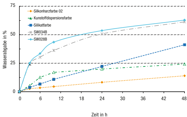
Abb. 1 // Rücktrocknungsverhalten unterschiedlicher Fassadenfarben.
