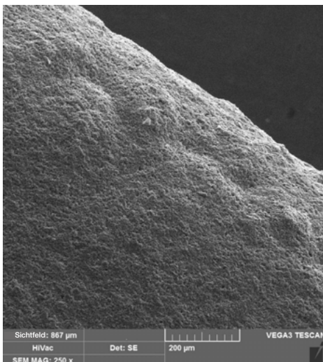
Abb. 2a-c // Oberflächenstrukturen von Fassadenfarben bei 250-facher Vergrößerung; links: Silikatfarbe, Mitte: funktionalisierte Acrylat-Dispersionsfarbe, rechts: Silikonharzfarbe.
