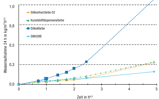
Abb. 3 // Bestimmung der kapillaren Wasseraufnahme nach DIN EN ISO 1062.
