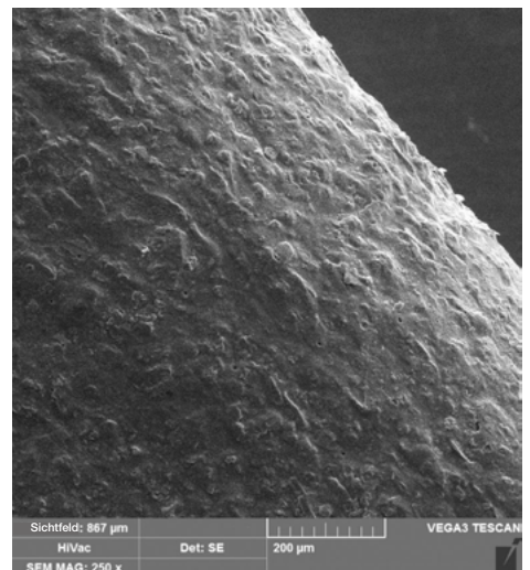
Abb. 2a-c // Oberflächenstrukturen von Fassadenfarben bei 250-facher Vergrößerung; links: Silikatfarbe, Mitte: funktionalisierte Acrylat-Dispersionsfarbe, rechts: Silikonharzfarbe.
